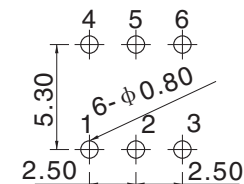
PCB Layout(Pattern Side)
