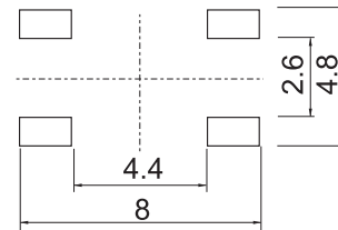
P.C.B.Land Pattern
