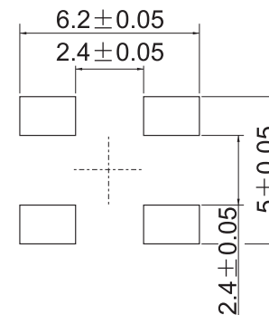
P.C.B.Land Pattern
