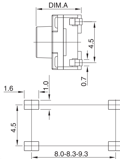
P.C.B PLACEMENT
