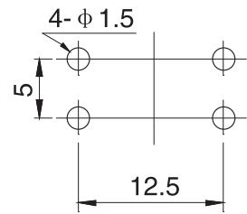
P.C.B.Land Pattern
