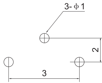
P.C.B.Land Pattern
