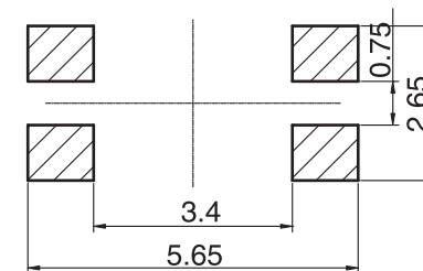
安装参考图
