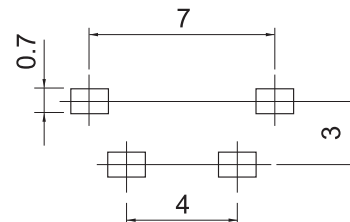
P.C.B.Land Pattern
