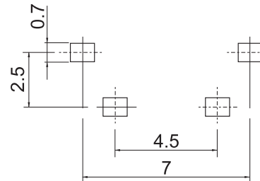
P.C.B.Land Pattern
