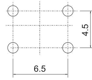
P.C.B.Land Pattern
